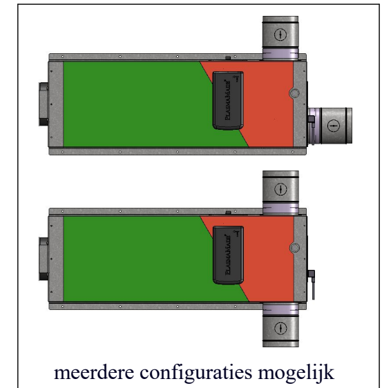
regelkleppen rond 125mm
